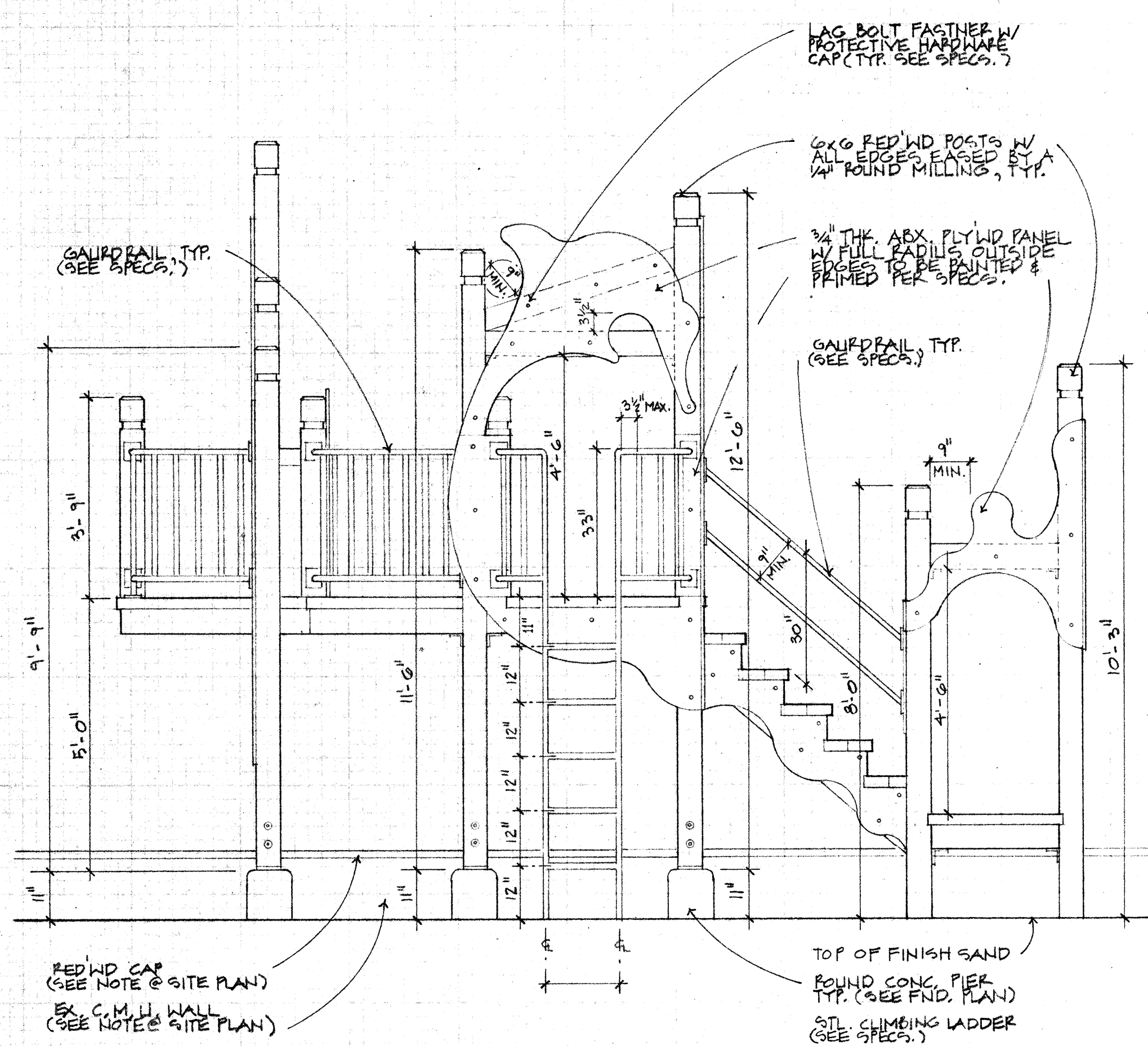
Elevation A
